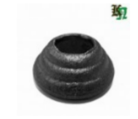
Основание балясины, арт. 7.348 д=40мм, отв.д=16мм Вес: 0.05 кг Цена: 49 руб.
